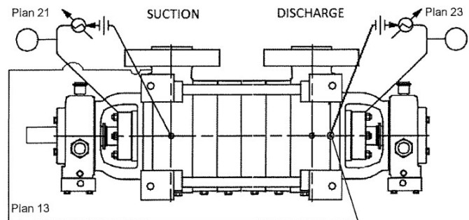
OPTIONAL PLAN 21/23/13
