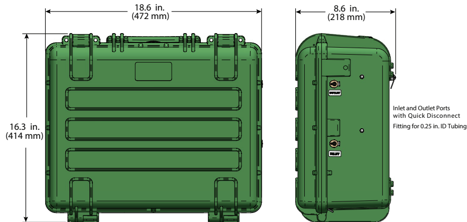
Figure 7: Mini portable case
