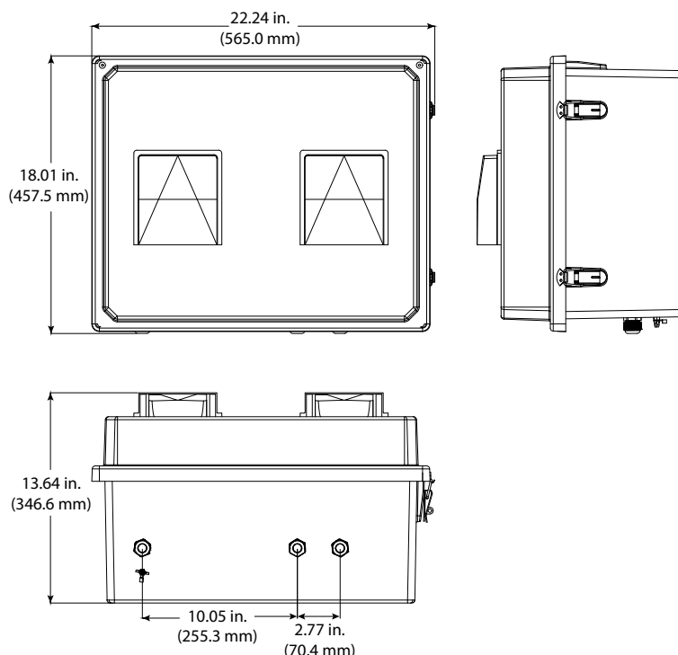
Figure 8: Mini fixed enclosure
